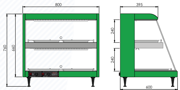
Bảng vẽ kỹ thuật
